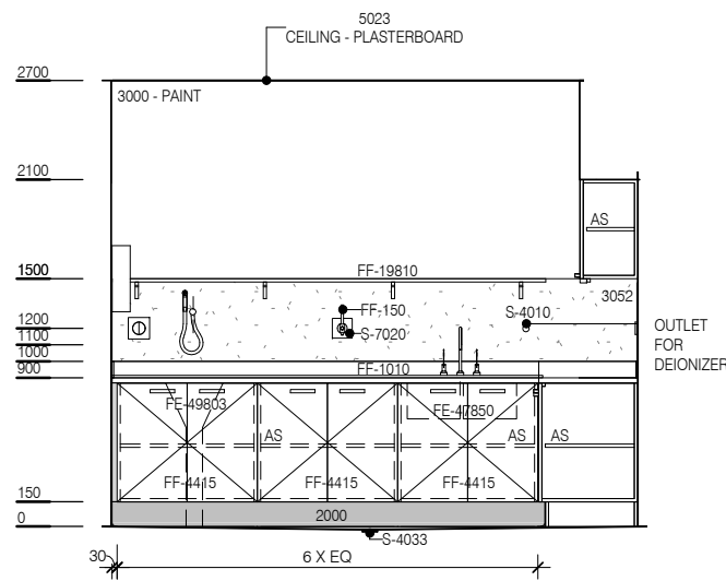
ELEVATION 1
