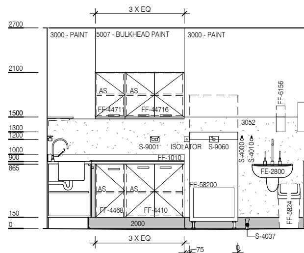
ELEVATION 2
