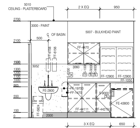
ELEVATION 4
