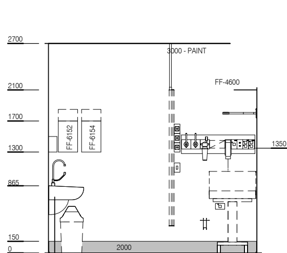
ELEVATION 1
