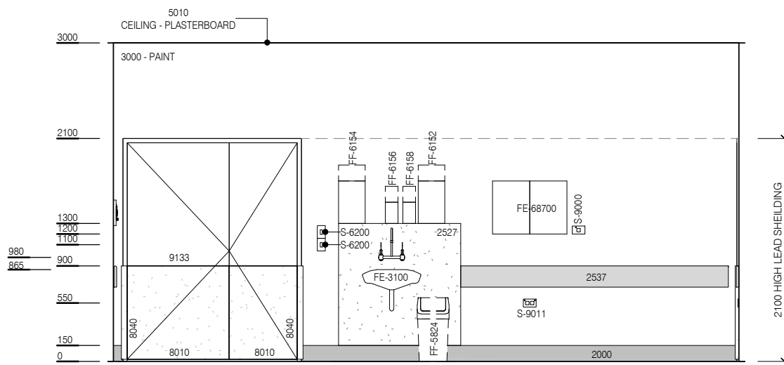
ELEVATION 3
