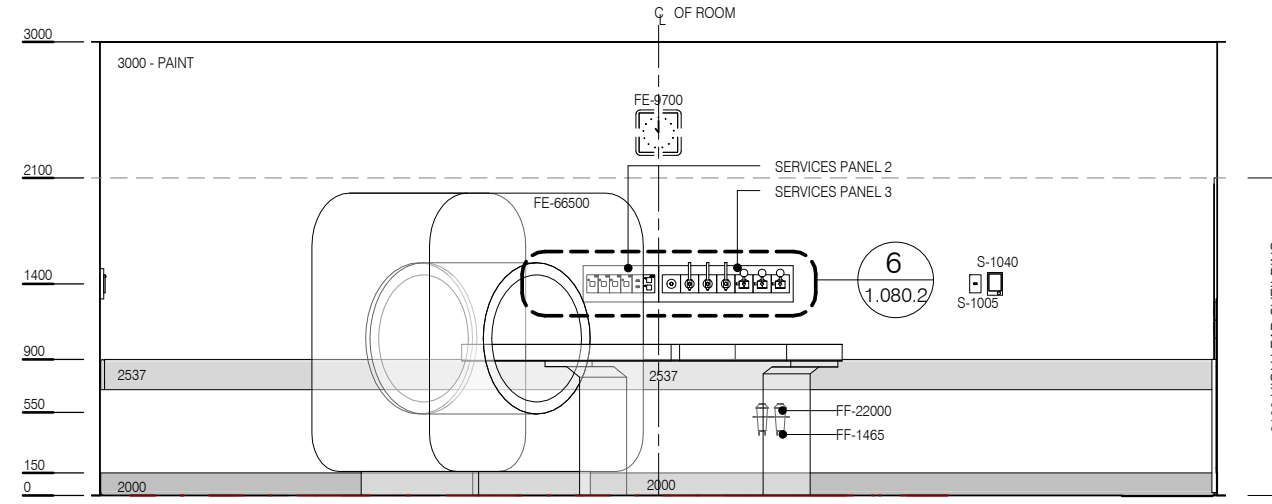
ELEVATION 2
