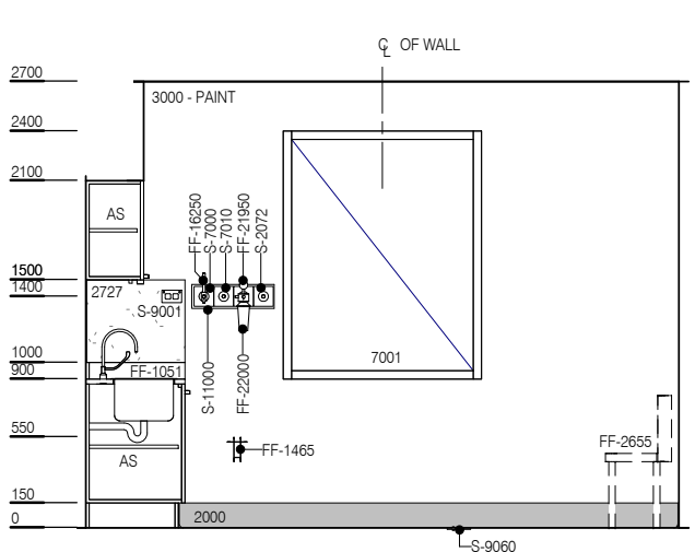
ELEVATION 1
