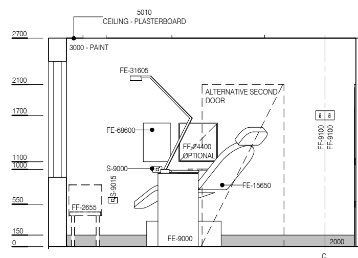
ELEVATION 2
