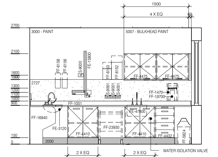
ELEVATION 4
