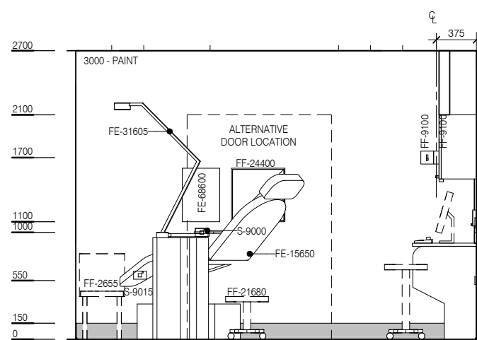
ELEVATION 2
