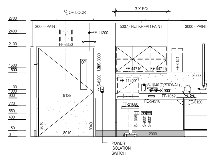
ELEVATION 3
