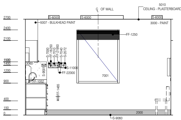
ELEVATION 1
