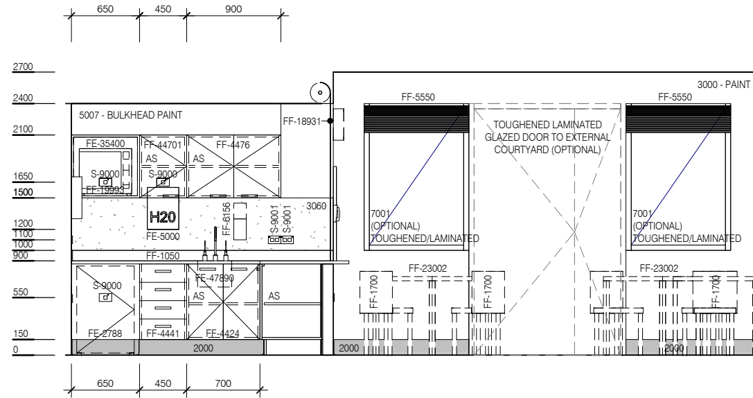
ELEVATION 1
