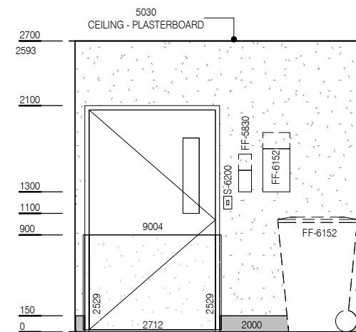
ELEVATION 3
