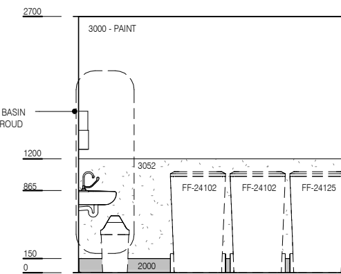
ELEVATION 4
