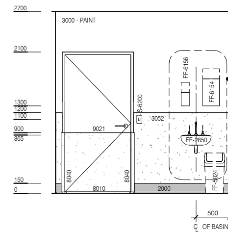
ELEVATION 3
