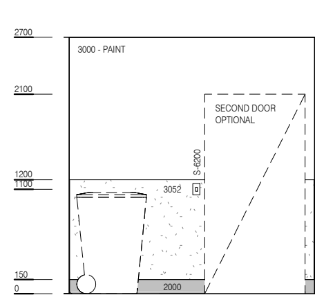
ELEVATION 1
