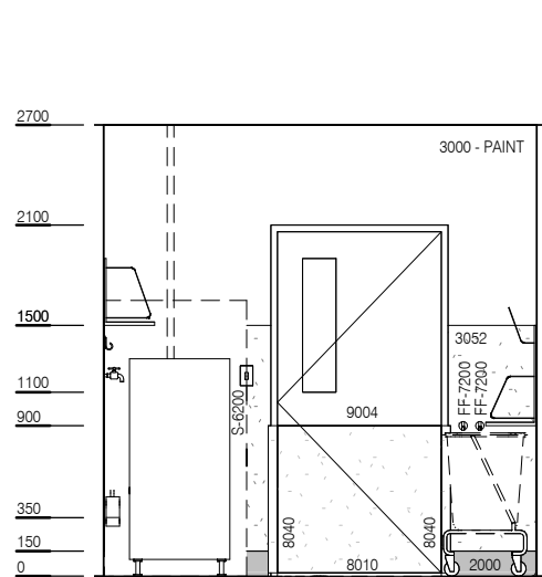
ELEVATION 1
