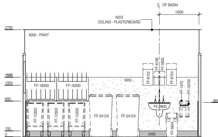
ELEVATION 2
