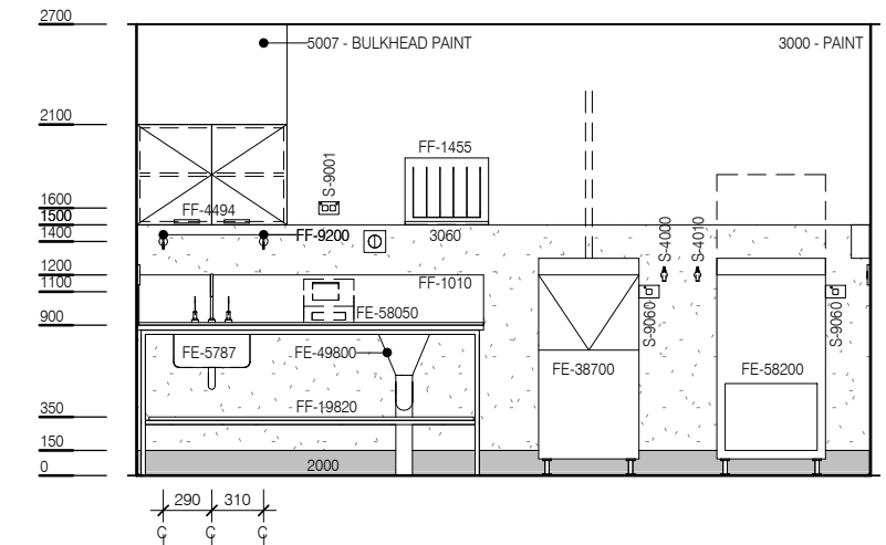
ELEVATION 4
