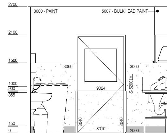
ELEVATION 3
