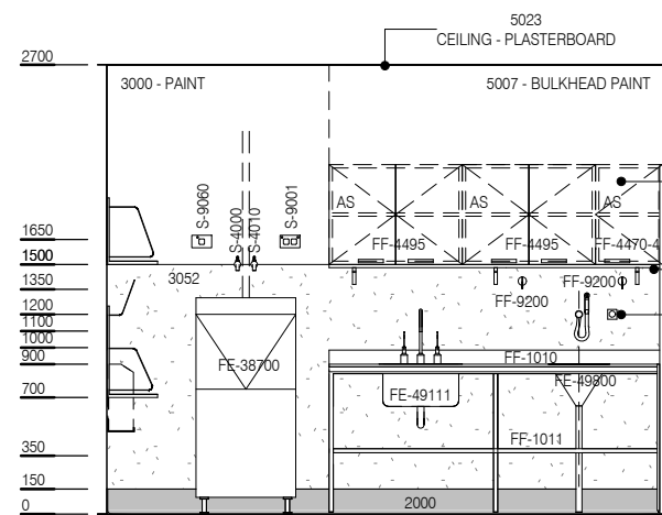
ELEVATION 2
