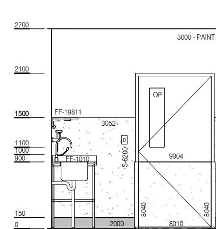
ELEVATION 3
