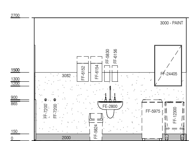
ELEVATION 4
