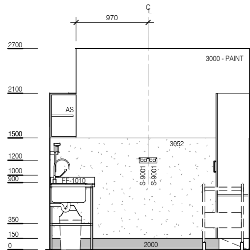
ELEVATION 1
