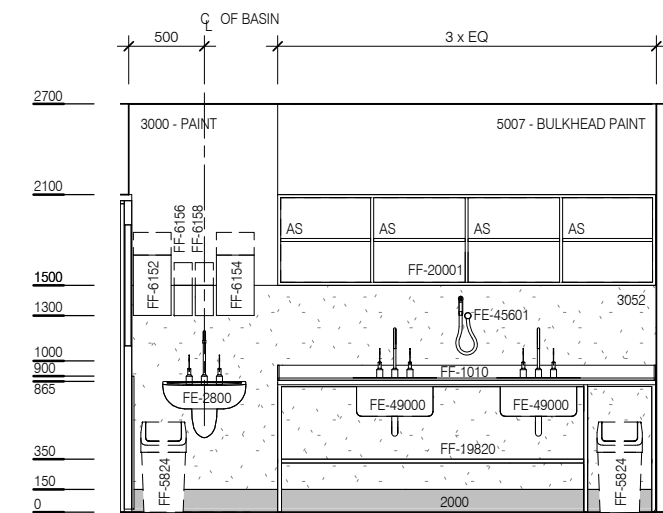
ELEVATION 4
