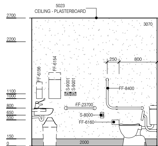
ELEVATION 2
