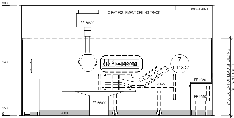
ELEVATION 2
