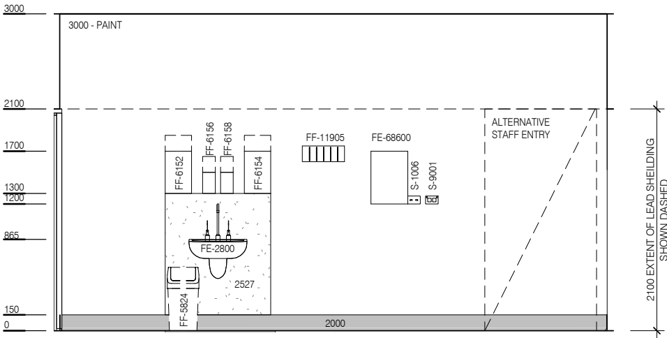
ELEVATION 4
