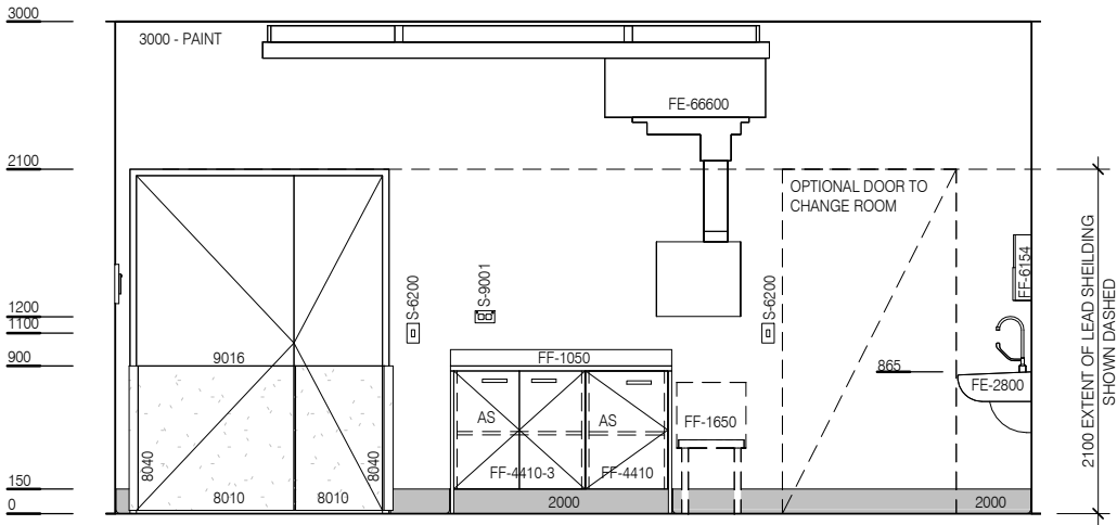
ELEVATION 3
