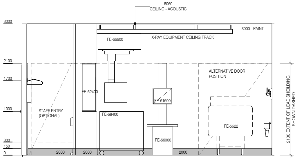
ELEVATION 1
