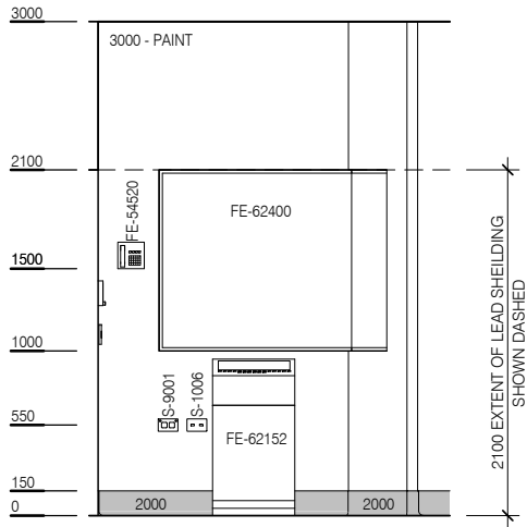
ELEVATION 5
