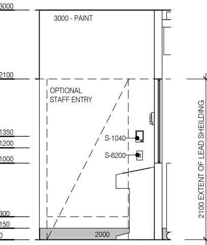
ELEVATION 6
