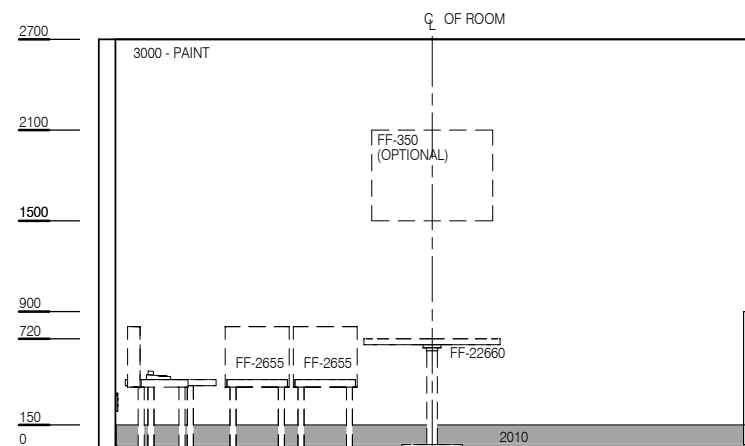
ELEVATION 2
