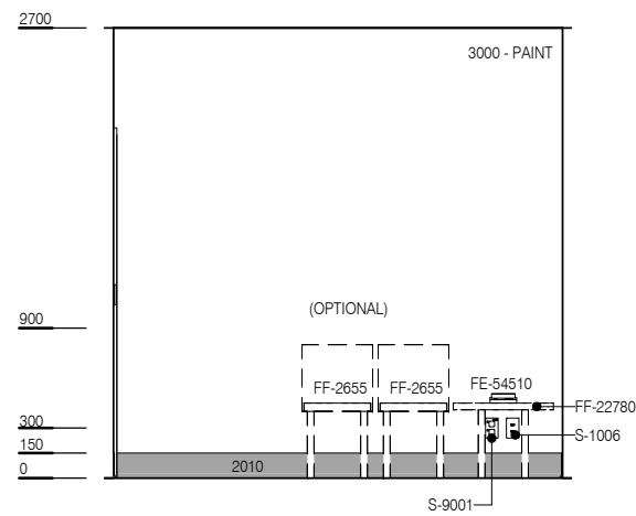
ELEVATION 1
