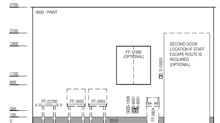
ELEVATION 4
