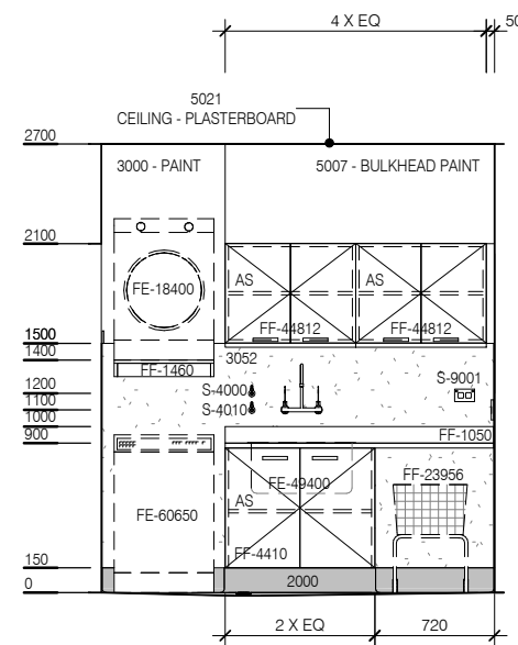
ELEVATION 2
