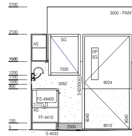
ELEVATION 3
