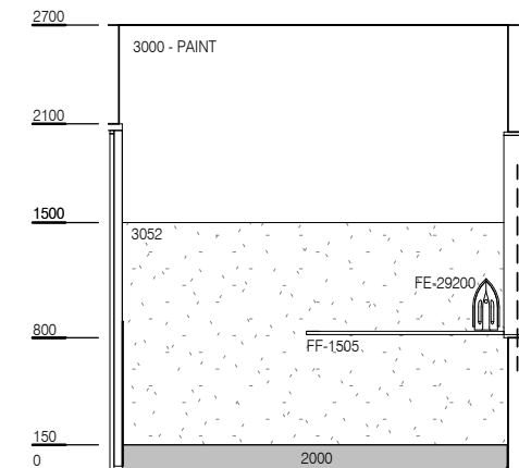
ELEVATION 4
