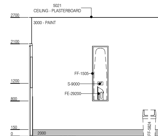
ELEVATION 4
