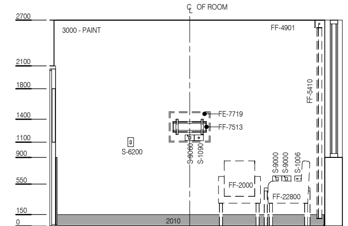
ELEVATION 4
