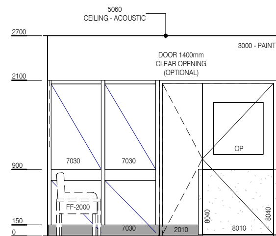
ELEVATION 3
