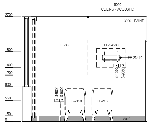
ELEVATION 2
