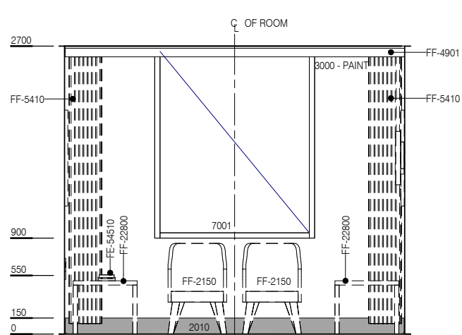
ELEVATION 1
