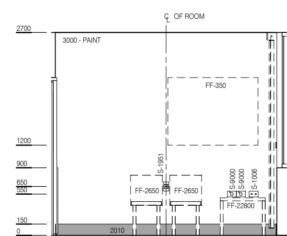
ELEVATION 4
