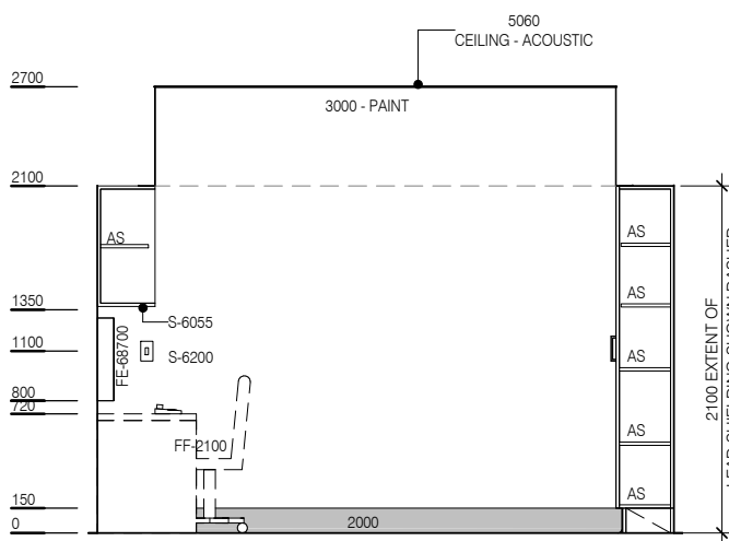
ELEVATION 1
