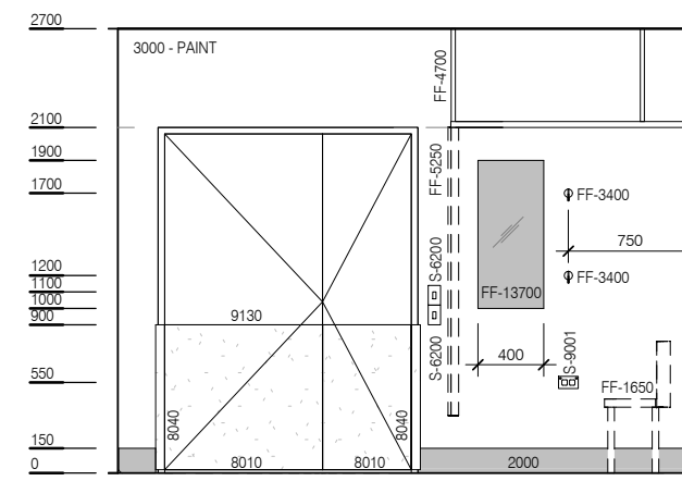
ELEVATION 3
