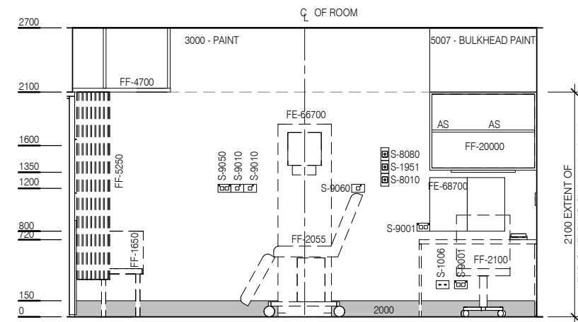
ELEVATION 4
