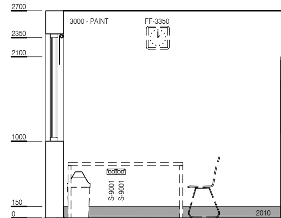
ELEVATION 2
