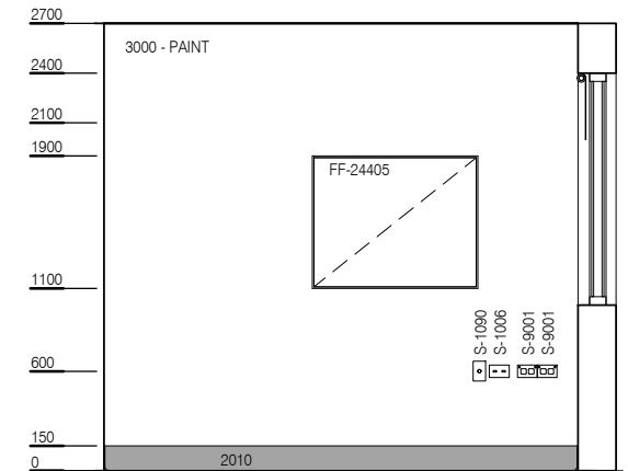
ELEVATION 4
