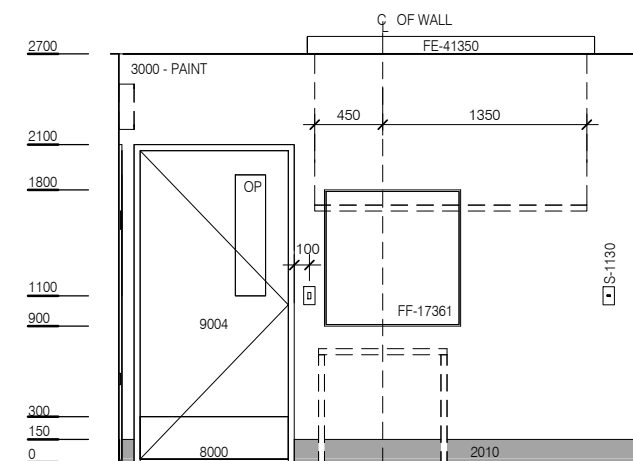
ELEVATION 3
