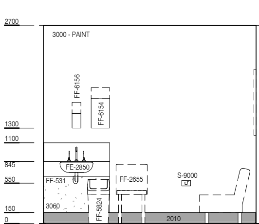
ELEVATION 3
