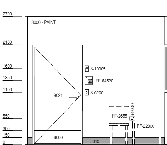
ELEVATION 1
