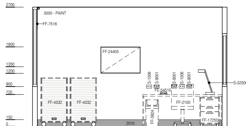
ELEVATION 2
