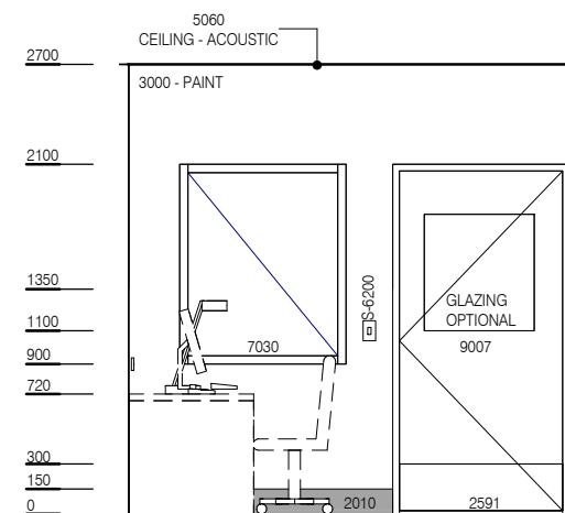
ELEVATION 3
