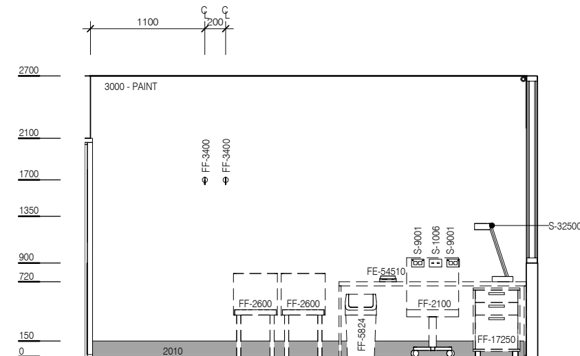
ELEVATION 4
