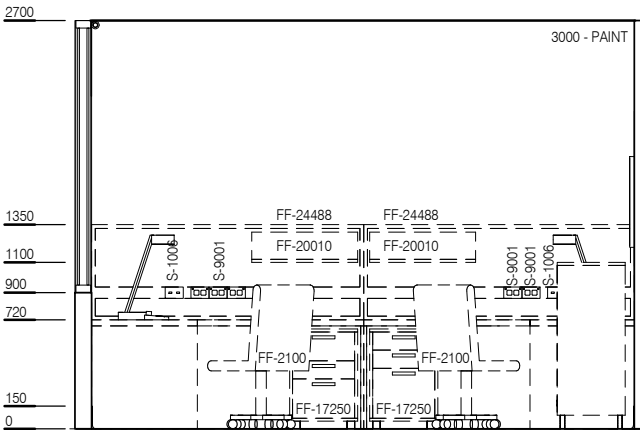
ELEVATION 2
