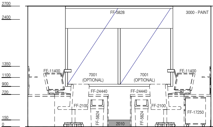
ELEVATION 1
