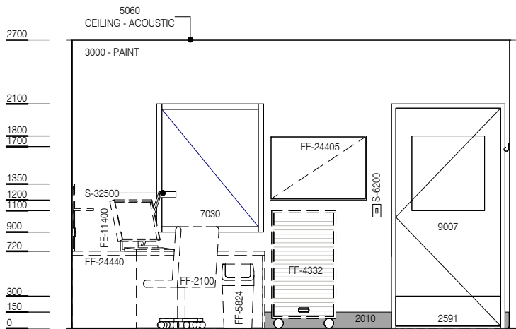
ELEVATION 3
