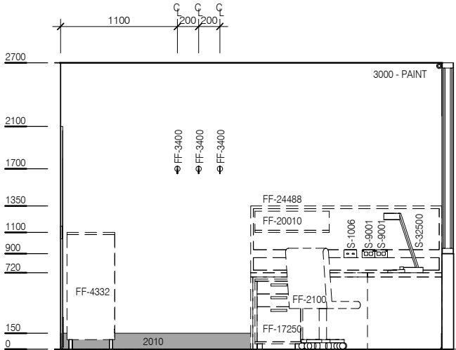
ELEVATION 4
