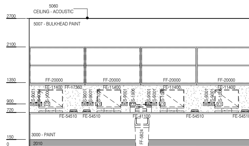
ELEVATION 2
