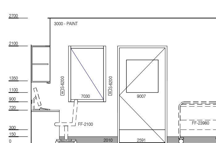
ELEVATION 3
