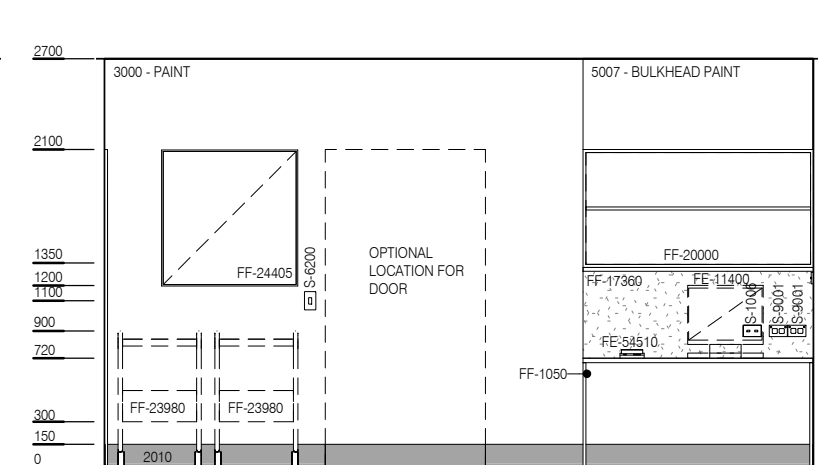
ELEVATION 4
