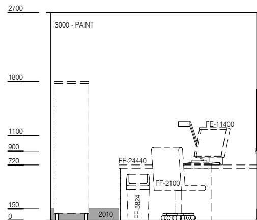
ELEVATION 1
