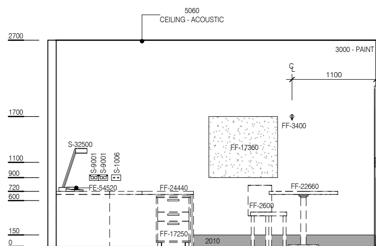
ELEVATION 2
