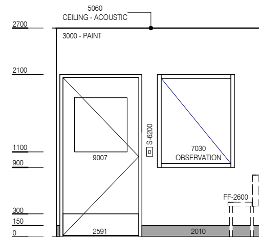
ELEVATION 3
