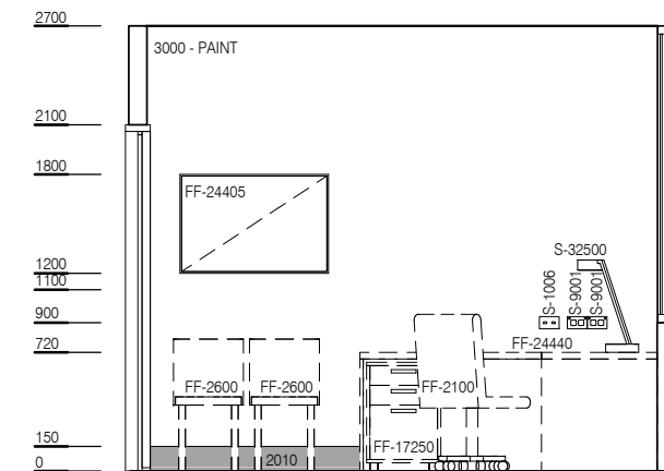
ELEVATION 4
