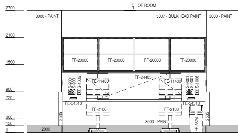
ELEVATION 2
