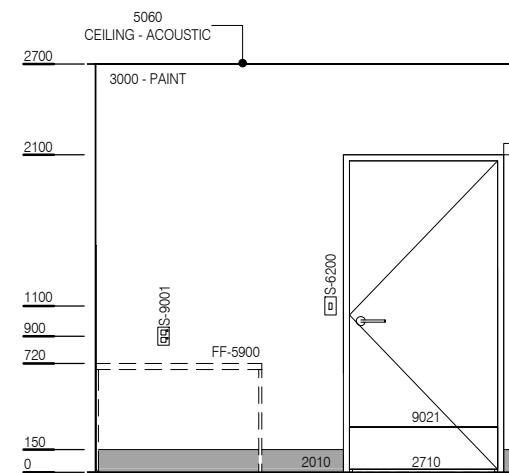
ELEVATION 3
