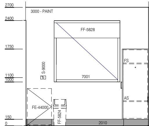
ELEVATION 1
