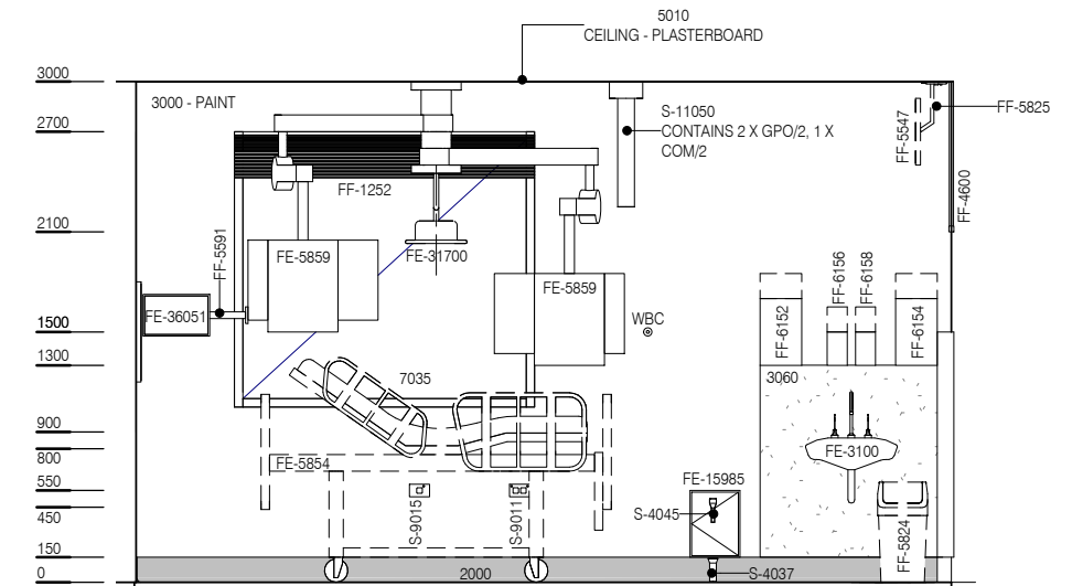
ELEVATION 2
