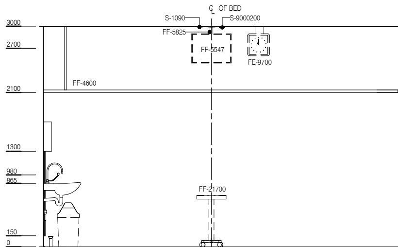
ELEVATION 3
