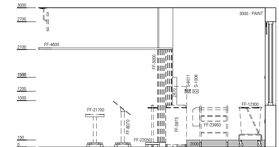
ELEVATION 4
