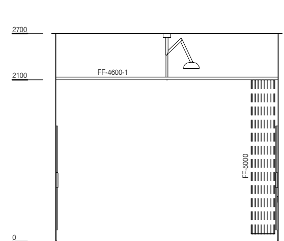
ELEVATION 3
