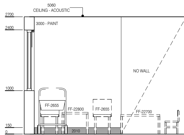
ELEVATION 2
