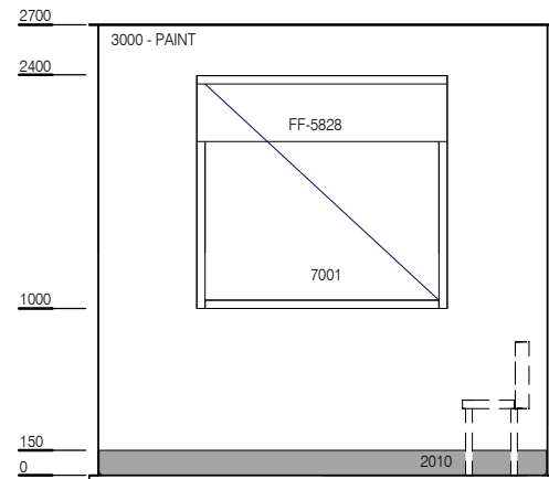
ELEVATION 1
