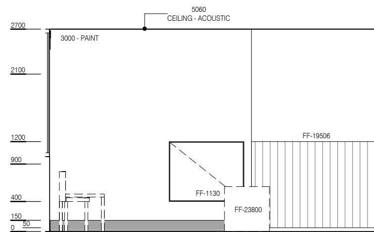
ELEVATION 2
