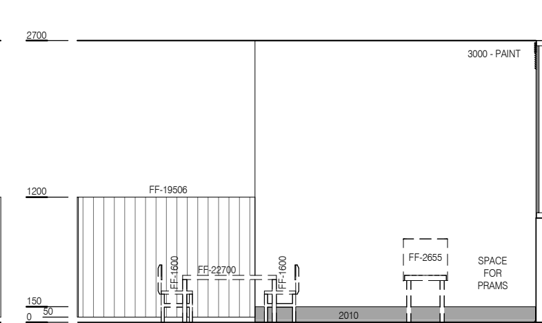
ELEVATION 4
