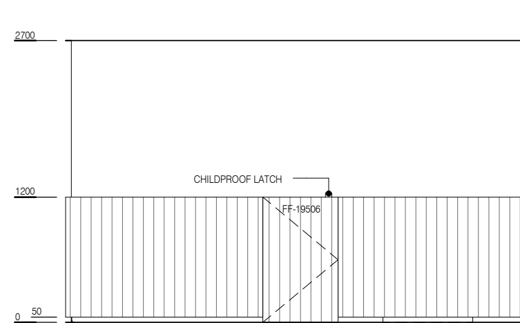
ELEVATION 3
