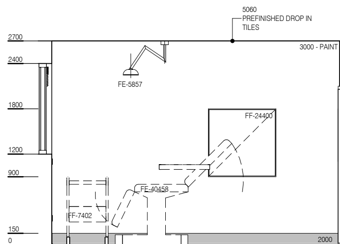
ELEVATION 2
