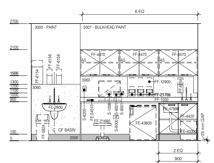
ELEVATION 4
