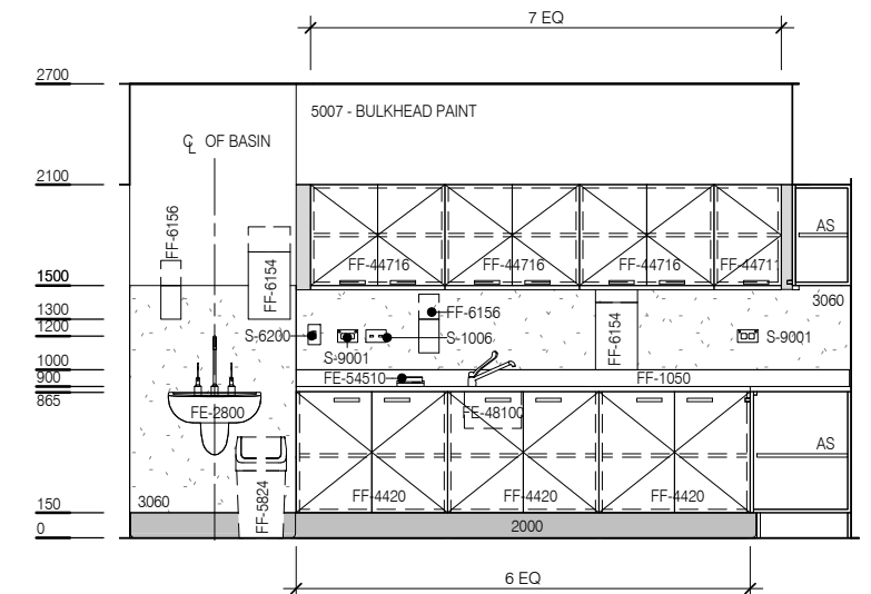
ELEVATION 4
