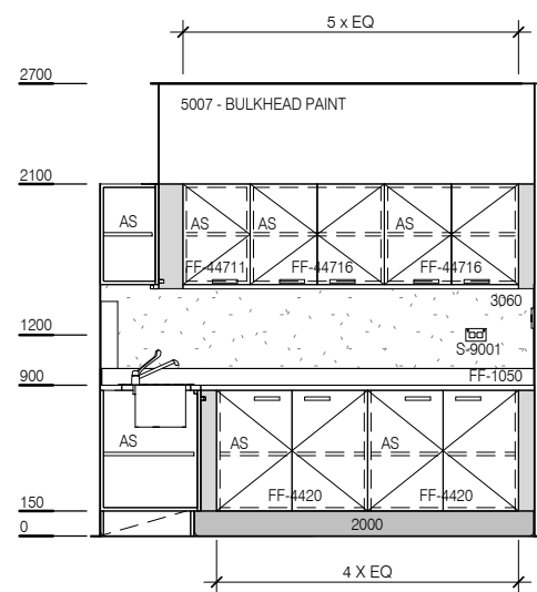
ELEVATION 1
