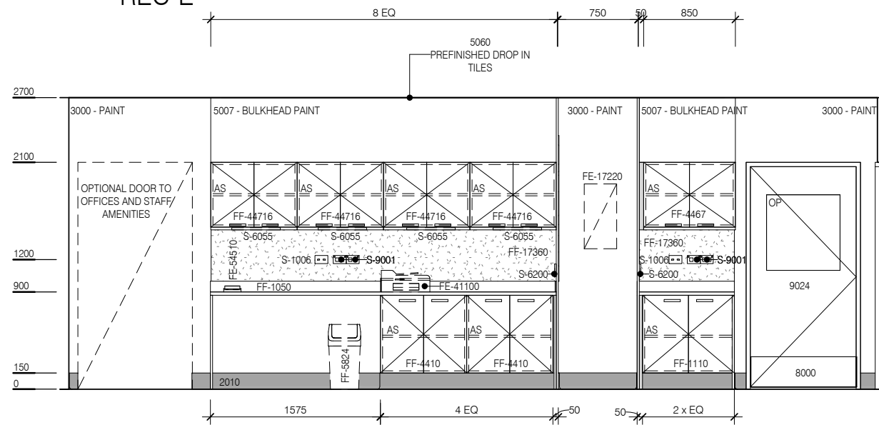
ELEVATION 1
