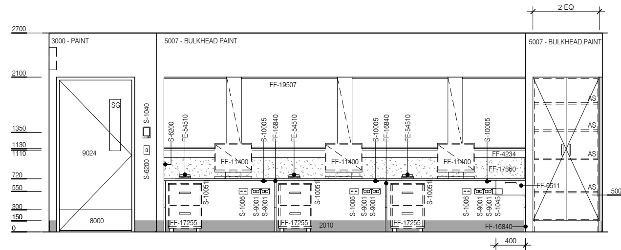
ELEVATION 3
