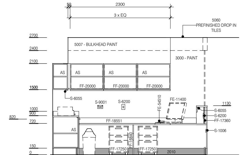
ELEVATION 6
