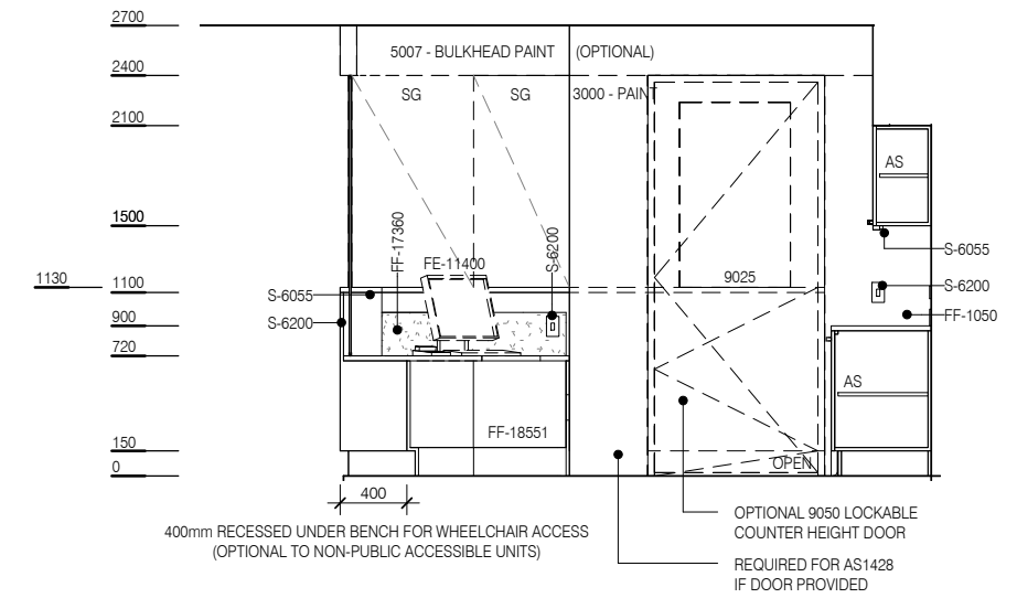
ELEVATION 4
