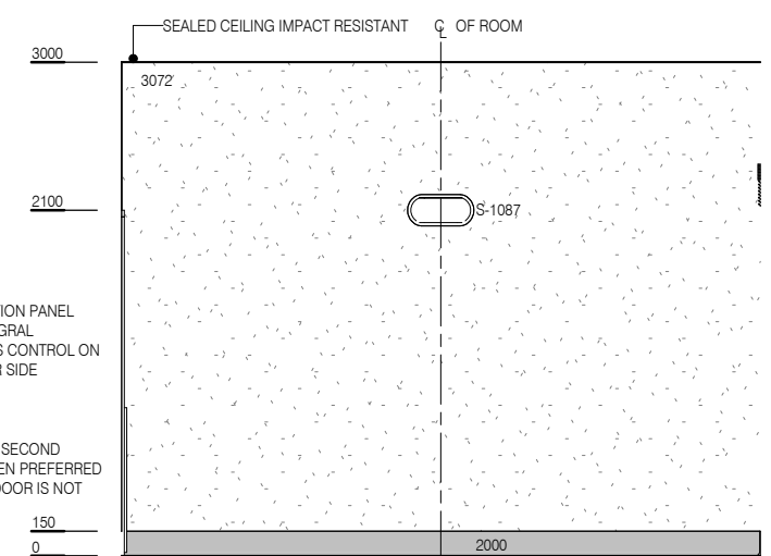
ELEVATION 4
