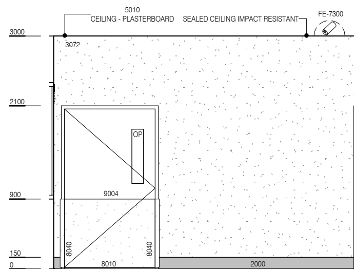
ELEVATION 2
