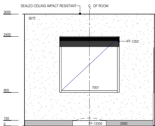
ELEVATION 1
