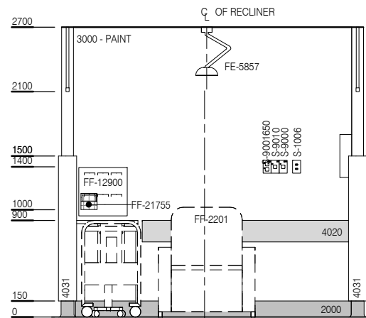
ELEVATION 1
