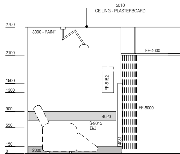
ELEVATION 2
