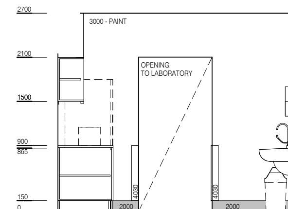
ELEVATION 2
