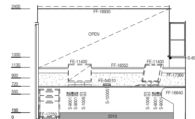
ELEVATION 4
