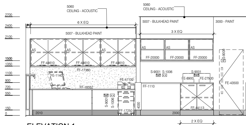
ELEVATION 1
