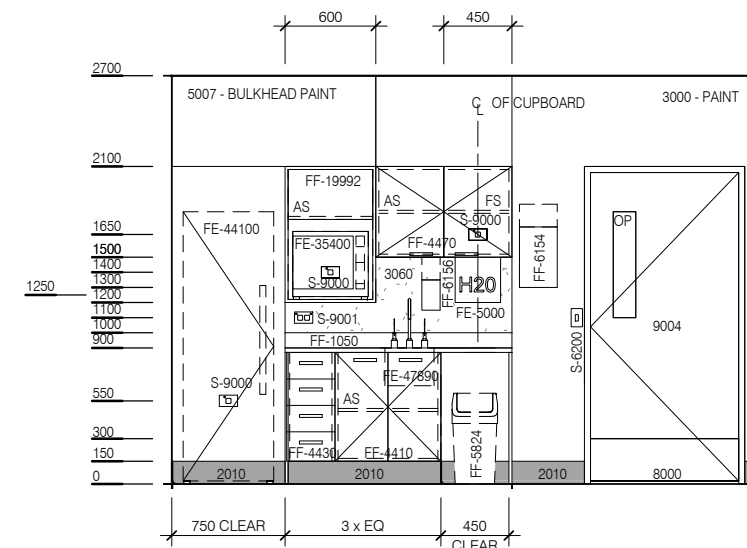
ELEVATION 3
