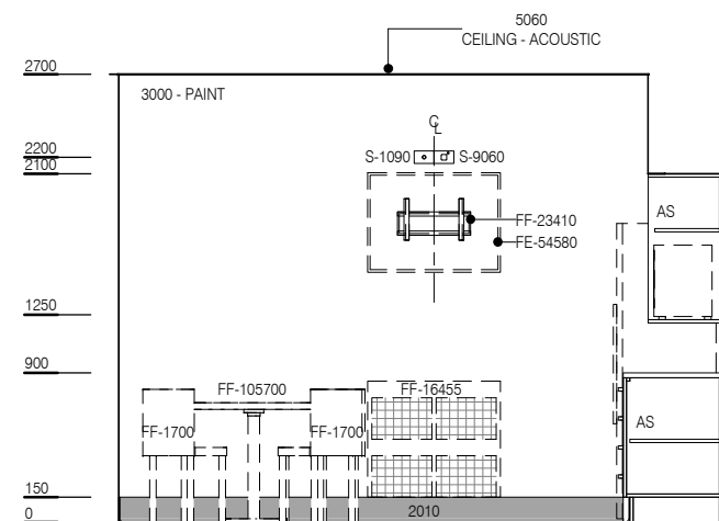
ELEVATION 2
