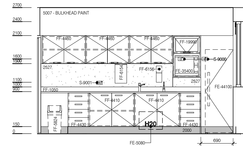
ELEVATION 4
