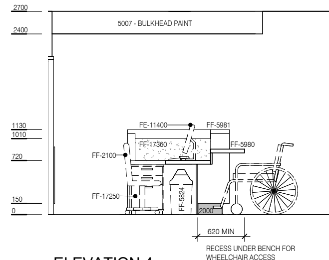
ELEVATION 4
