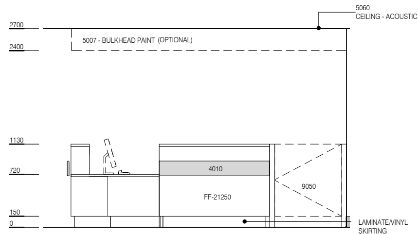
ELEVATION 1
