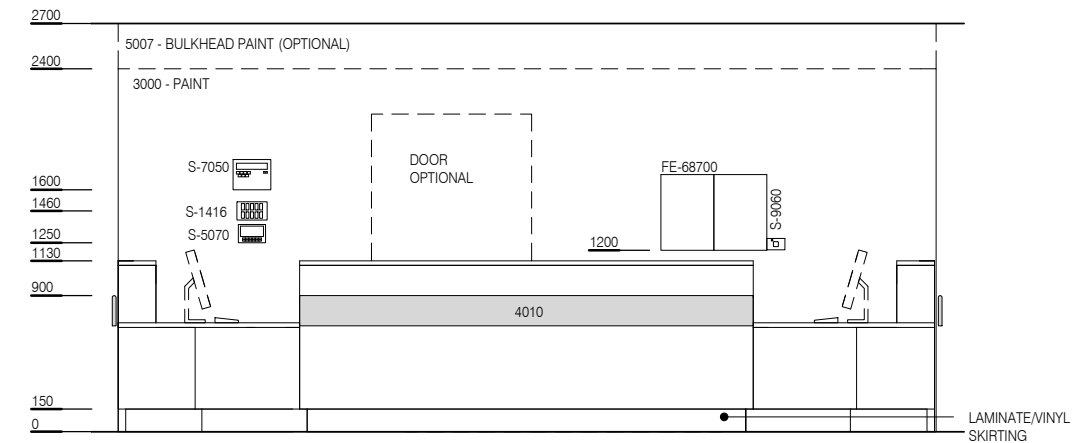
ELEVATION 2
