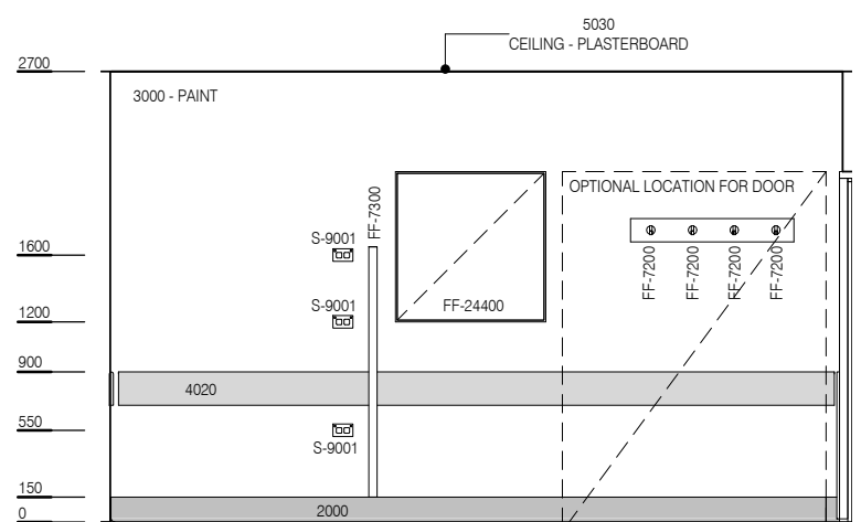
ELEVATION 2
