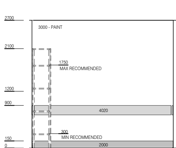
ELEVATION 1
