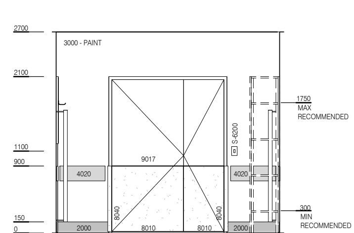
ELEVATION 3
