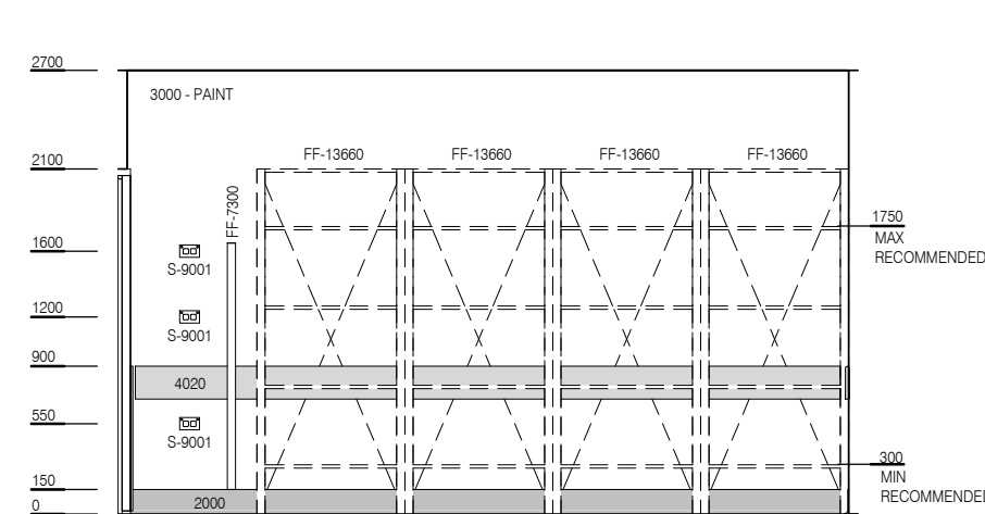
ELEVATION 4
