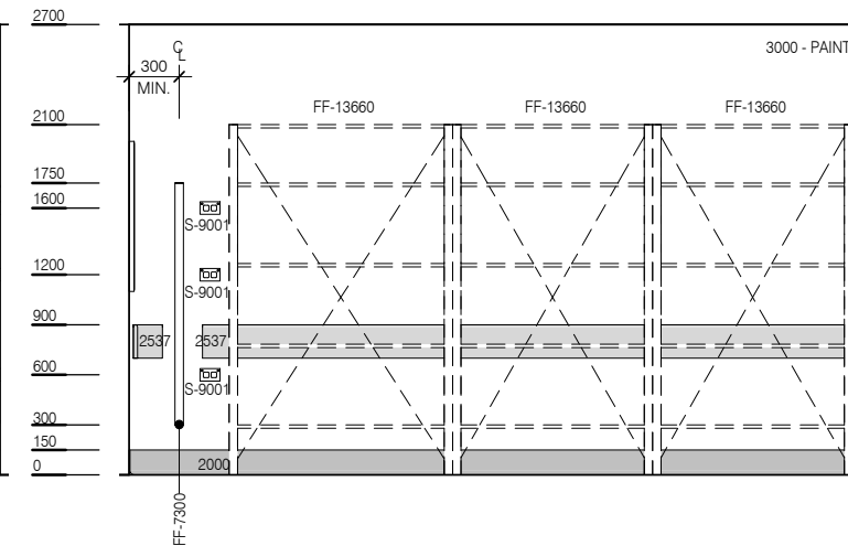
ELEVATION 4
