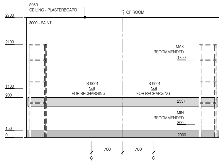
ELEVATION 1
