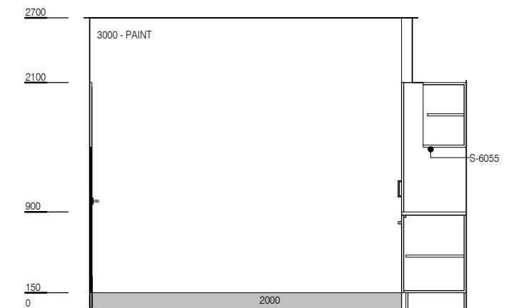
ELEVATION 4
