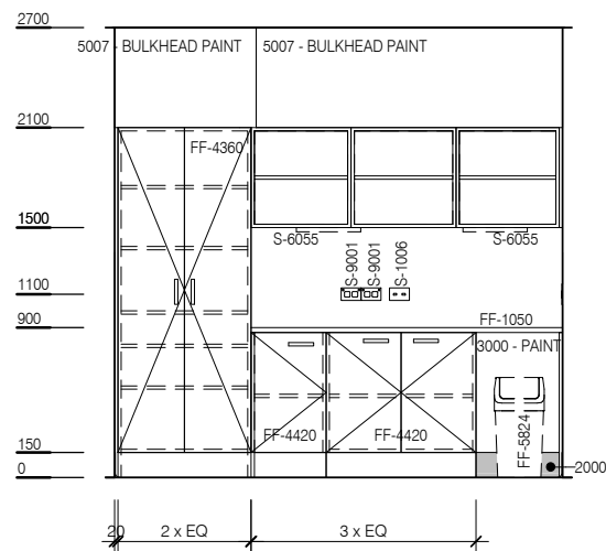
ELEVATION 1
