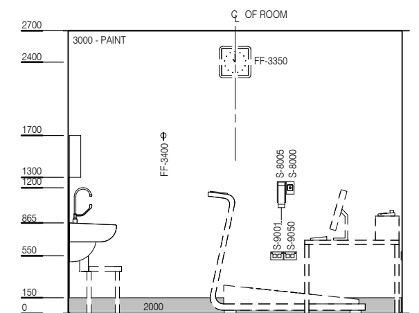
ELEVATION 4
